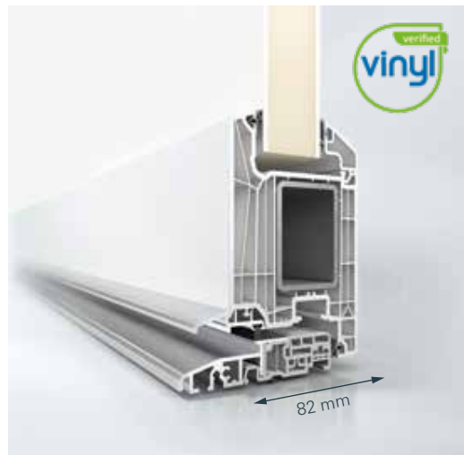
Haustürsystem Schüco Living
